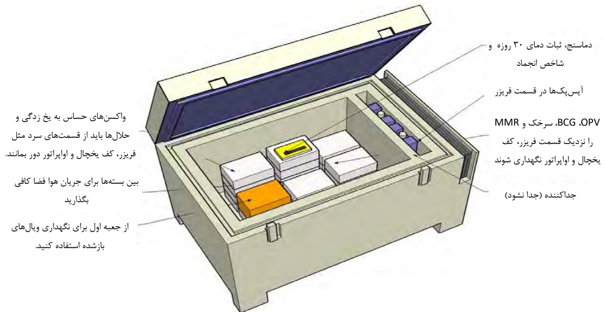
شکل ۲- یخچال صندوقی
